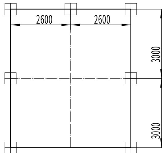
预埋件布置图
